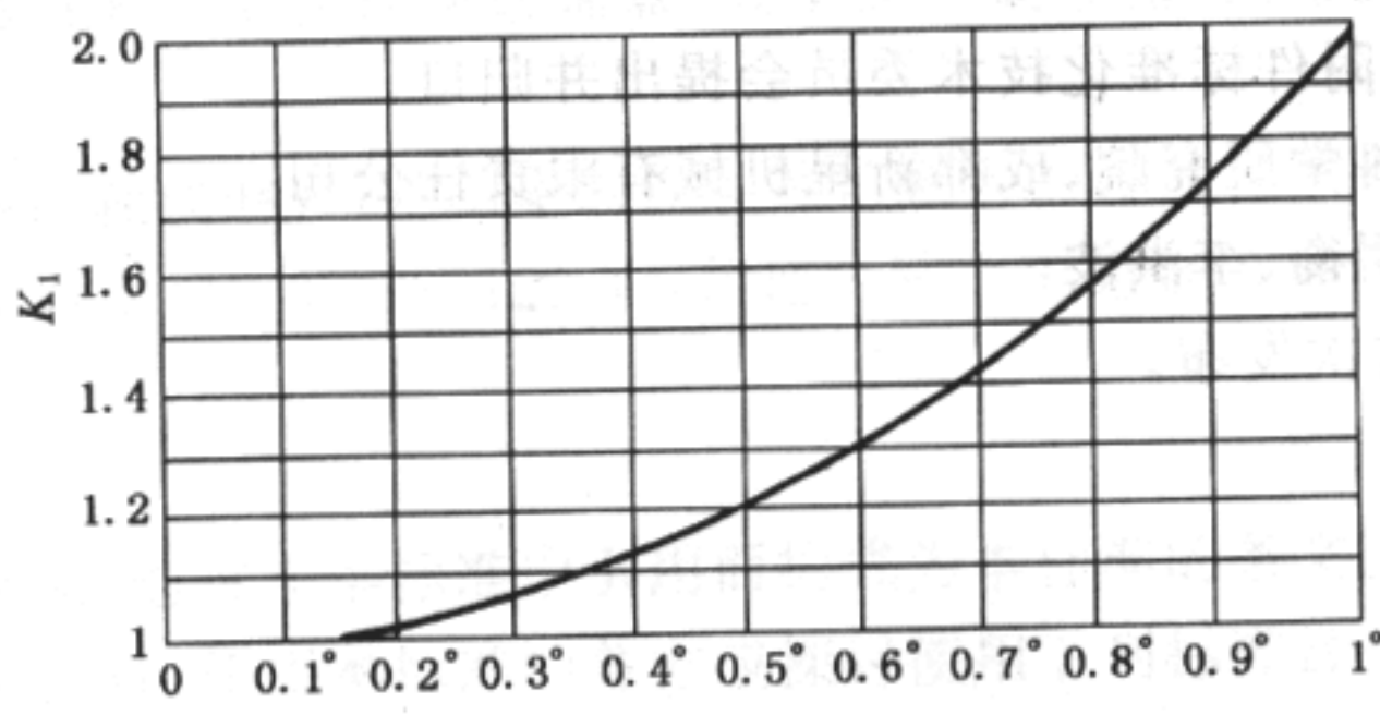
图 A1 轴线偏角
